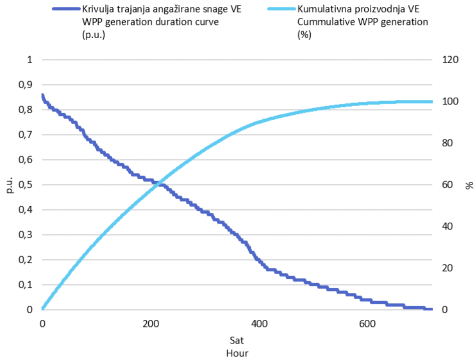
Slika 3 Krivulja trajanja angažirane snage svih VE i kumulativna proizvodnja VE u studenom 2022. godine u jediničnim vrijednostima
