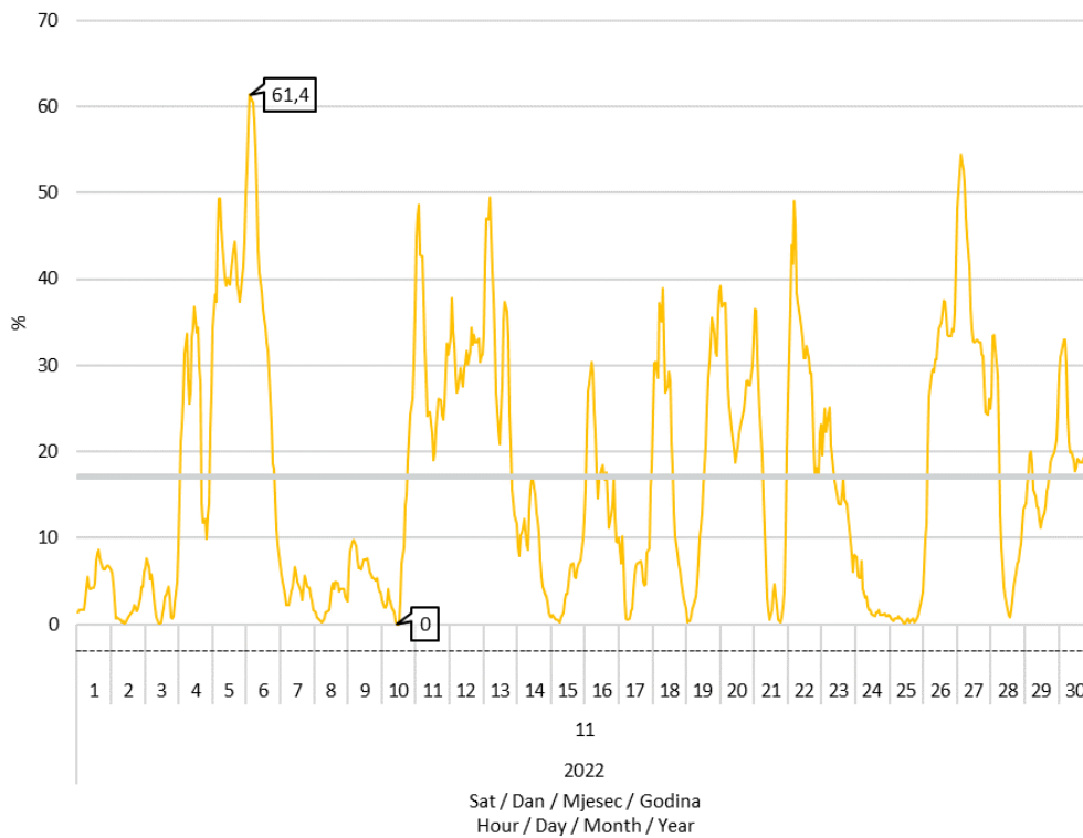
Slika 8 Udio proizvodnje vjetroelektrana u pokrivanju satnog opterećenja elektroenergetskog sustava u studenom 2022. godine
