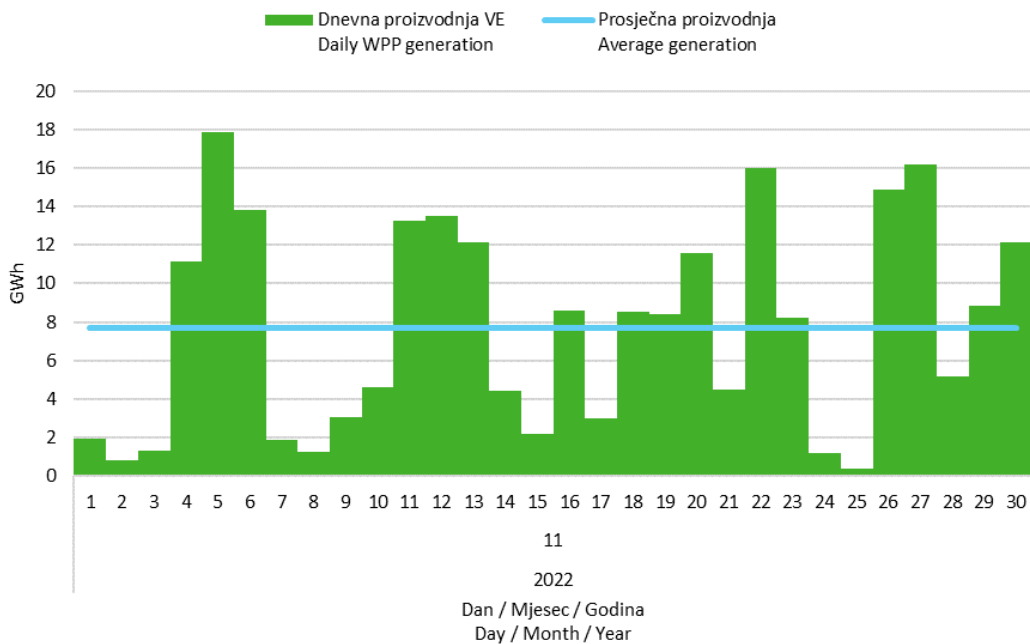
Slika 5 Dnevna proizvodnja svih vjetroelektrana u studenom 2022. godine Figure 5 Daily generation of all wind power plants in November 2022
