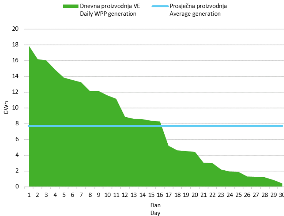
Slika 6 Krivulja trajanja dnevne proizvodnje vjetroelektrana u studenom 2022. godine
