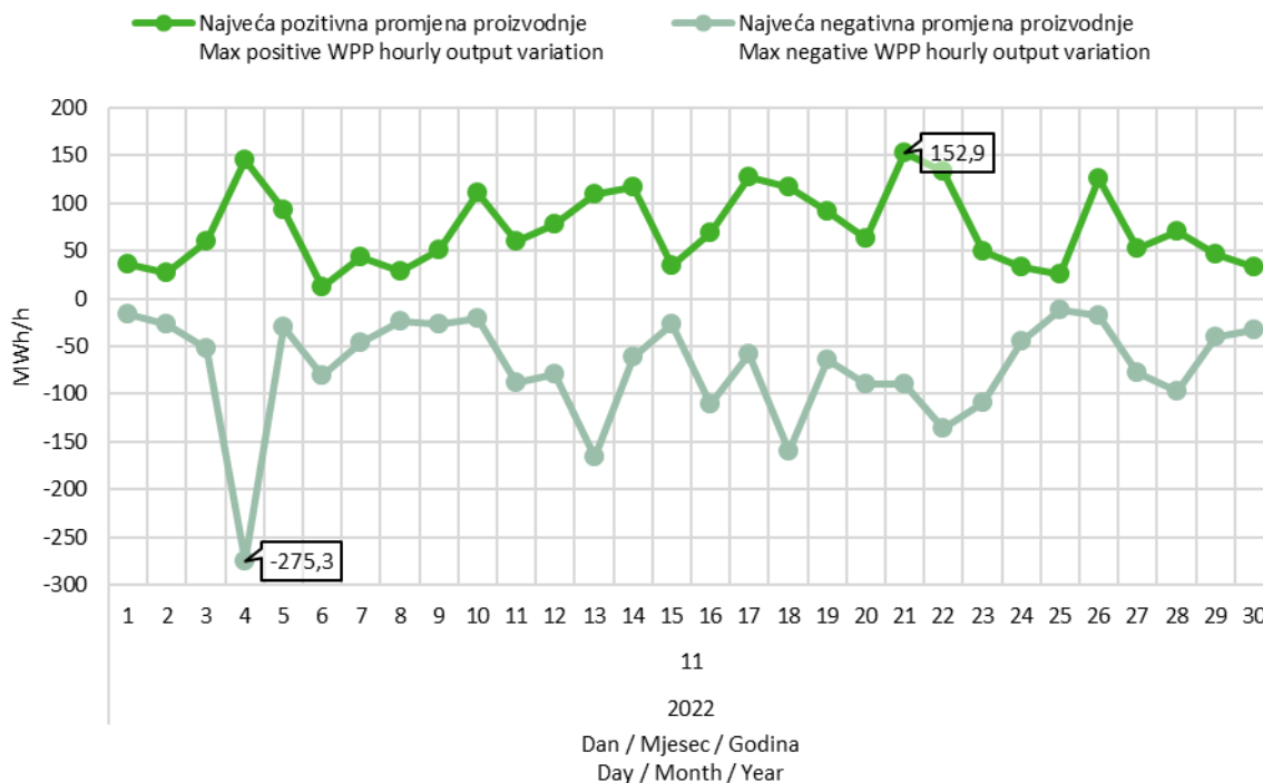
Slika 9 Maksimalna pozitivna i maksimalna negativna promjena satne proizvodnje VE u studenom 2022. godine
