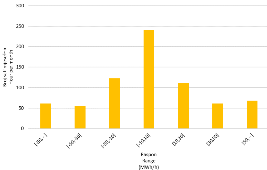
Slika 10 Statistička raspodjela satnih promjena proizvodnje VE u studenom 2022. godine
