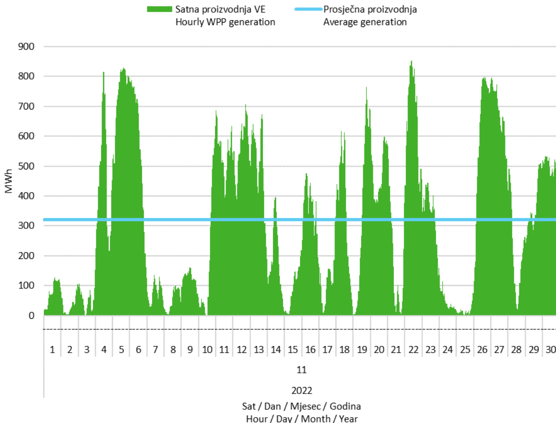
Slika 2 Satna proizvodnja svih vjetroelektrana u studenom 2022. godine
